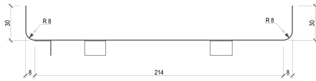
NÁRYS - 1:2
