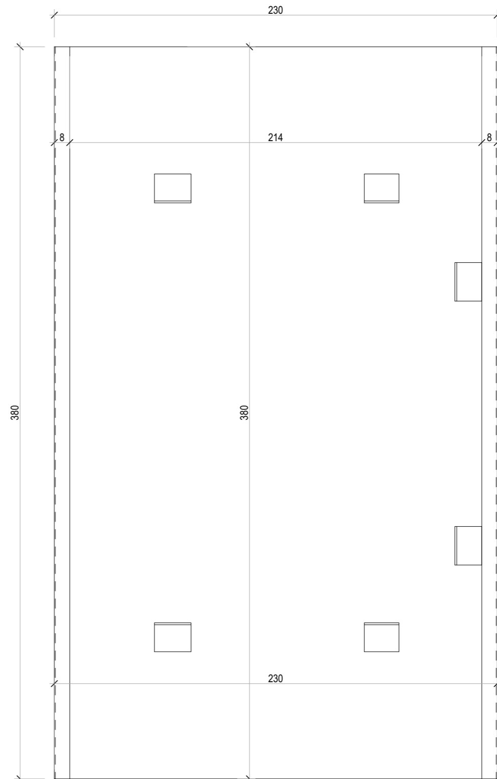
PŮDORYS (ZE SPODU) - 1:2
